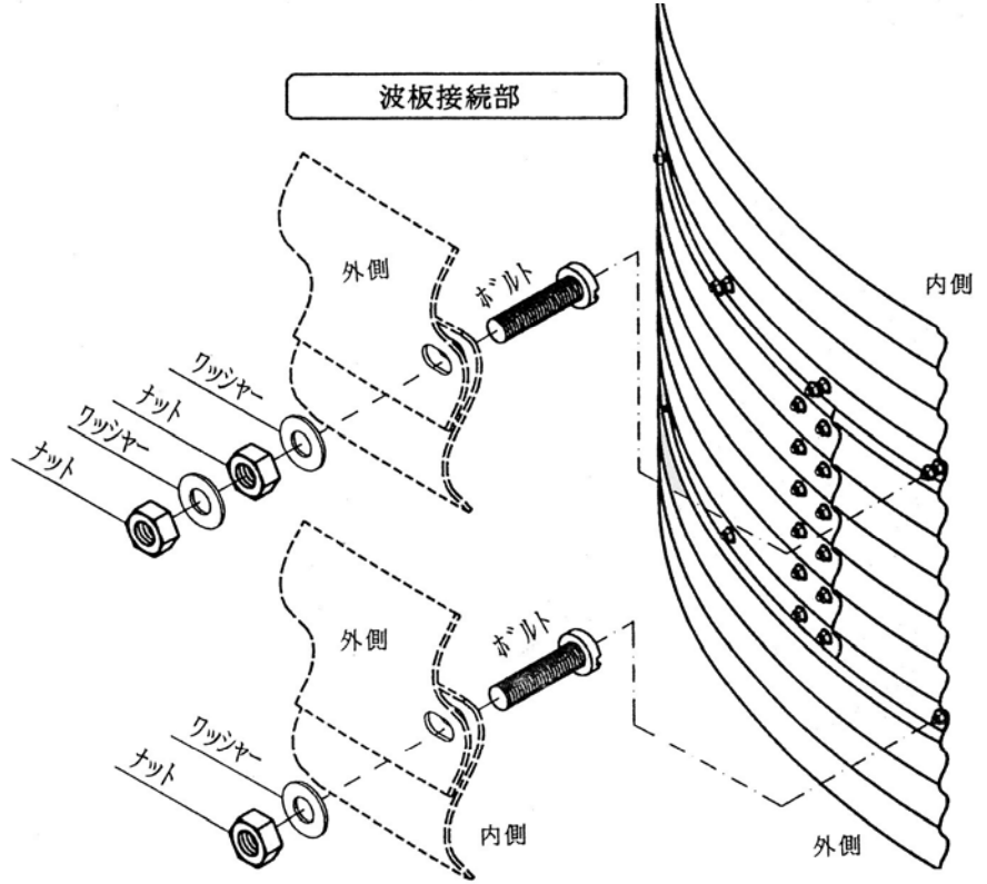
波板詳細図
