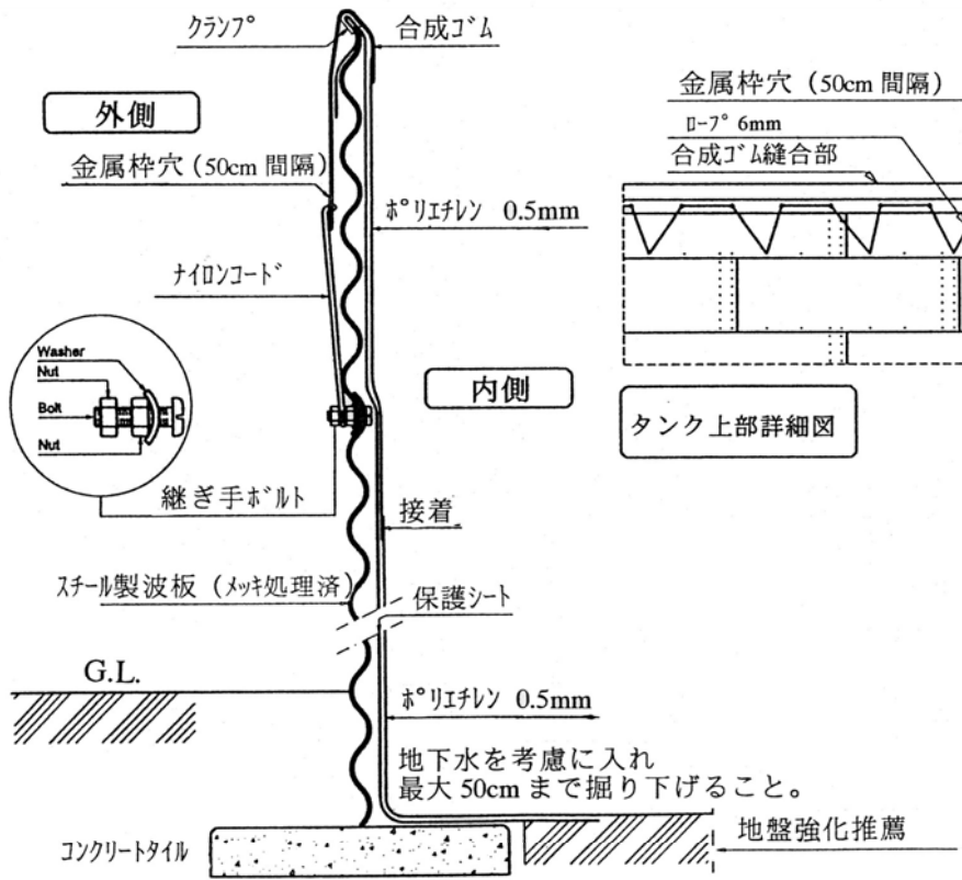
タンク側面図
