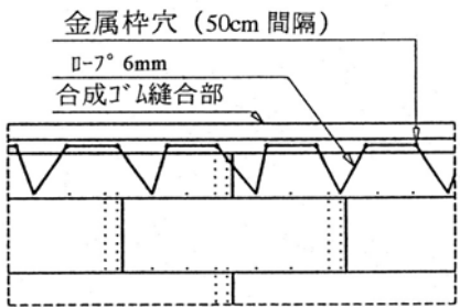
タンク上部詳細図
